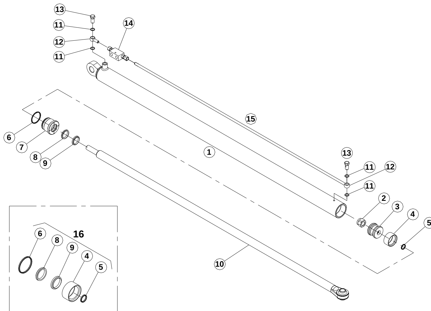
Tavola 14 - Table 14 - Planche 14 - EASY RAKE SUPER STAR 16-18-20 AUTOSTERZ.-AUTOSTEER-AUTODIRECTEUR
