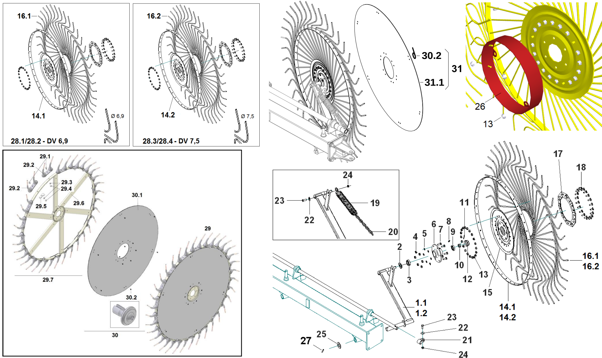
Tavola 13 - Table 13 - Planche 13 - EASY RAKE SUPER STAR 16-18-20 AUTOSTERZ.-AUTOSTEER-AUTODIRECTEUR (1/2)
