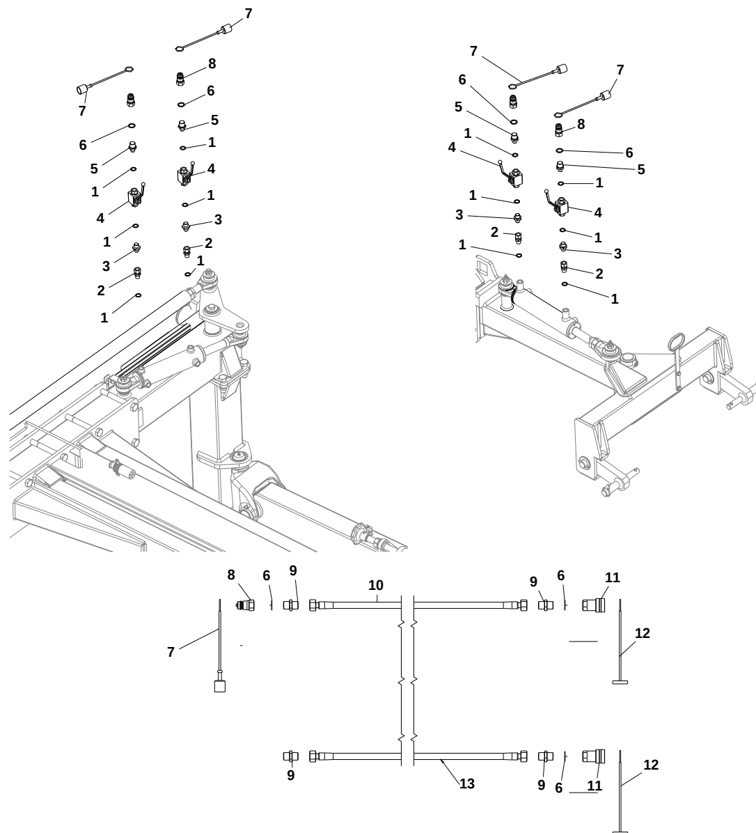
Tavola 26 - Table 26 - Planche 26 EASY RAKE SUPER STAR 16-18-20 AUTOSTERZ.-AUTOSTEER-AUTODIRECTEUR
