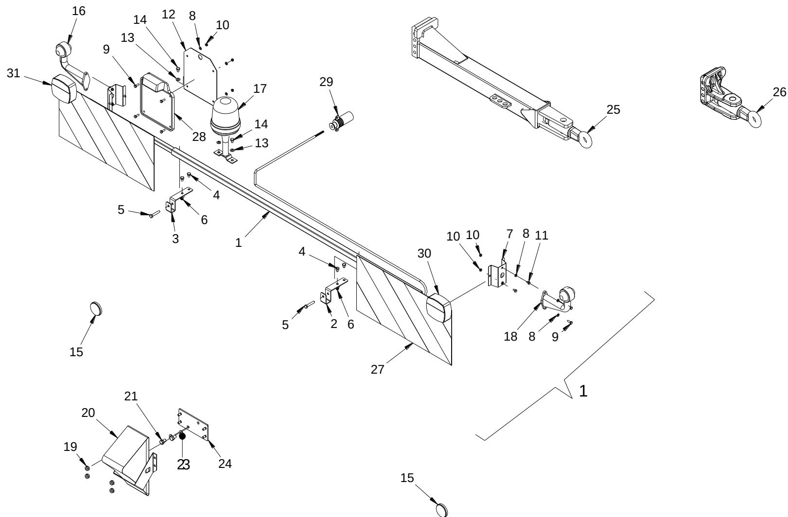
Tavola 18-Table 18-Planche 18 EASY RAKE SUPER STAR 16-18-20 / EASY RAKE SUPER STAR 16-18-20-22 AUTOSTERZ.-AUTOSTEER-AUTODIRECTEUR (OPTIONAL) – KIT LUCI PER OMOLOGAZIONE ITA-KIT LIGHT ITA-KIT LUMIERE ITA
