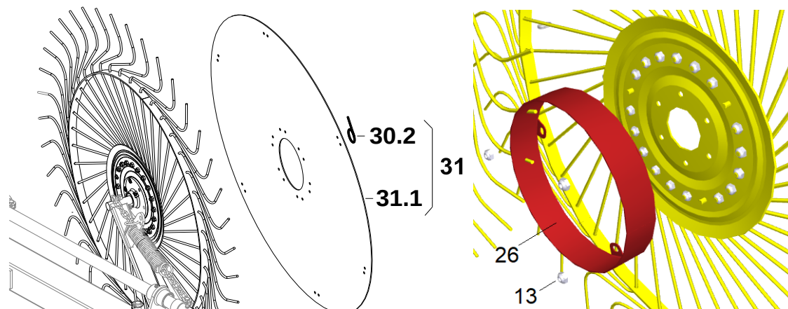
Tavola 13 - Table 13 - Planche 13 - EASY RAKE SUPER STAR 16-18-20 AUTOSTERZ.-AUTOSTEER-AUTODIRECTEUR (2/2)
