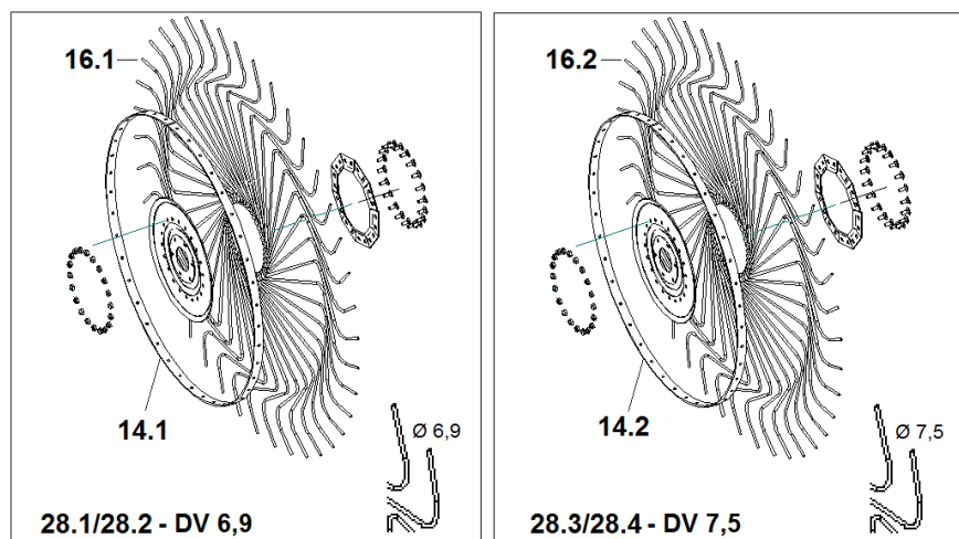
Tavola 13 - Table 13 - Planche 13 - EASY RAKE SUPER STAR 16-18-20 AUTOSTERZ.-AUTOSTEER-AUTODIRECTEUR (2/2)
