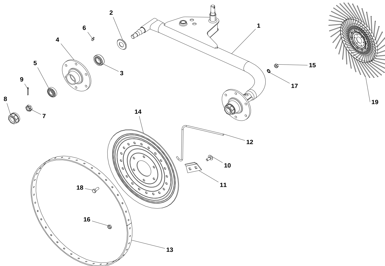
Tavola 15 - Table 15 - Planche 15 (OPTIONAL) - EASY RAKE SUPERSTAR 16-18-20 AUTOSTERZ.-AUTOSTEER-AUTODIRECTEUR
