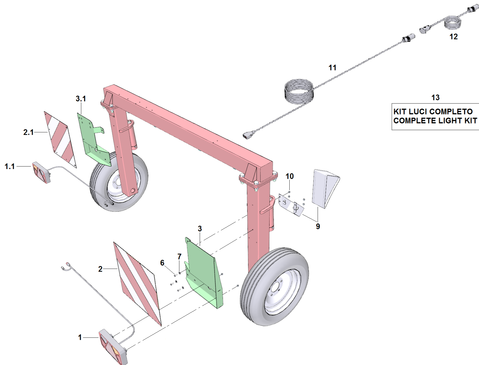
Tavola 17-Table 17-Planche 17 - (OPTIONAL) -EASY RAKE SUPER STAR 16-18-20 / EASY RAKE SUPER STAR 16-18-20-22 AUTOSTERZ.-AUTOSTEER-AUTODIRECTEUR – kit luci per circolazione stradale
