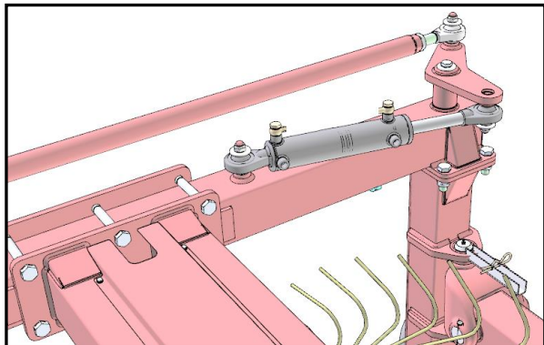
Tavola 25 - Table 25 - Planche 25 EASY RAKE SUPER STAR 16-18-20-22 AUTOSTERZ.-AUTOSTEER-AUTODIRECTEUR
