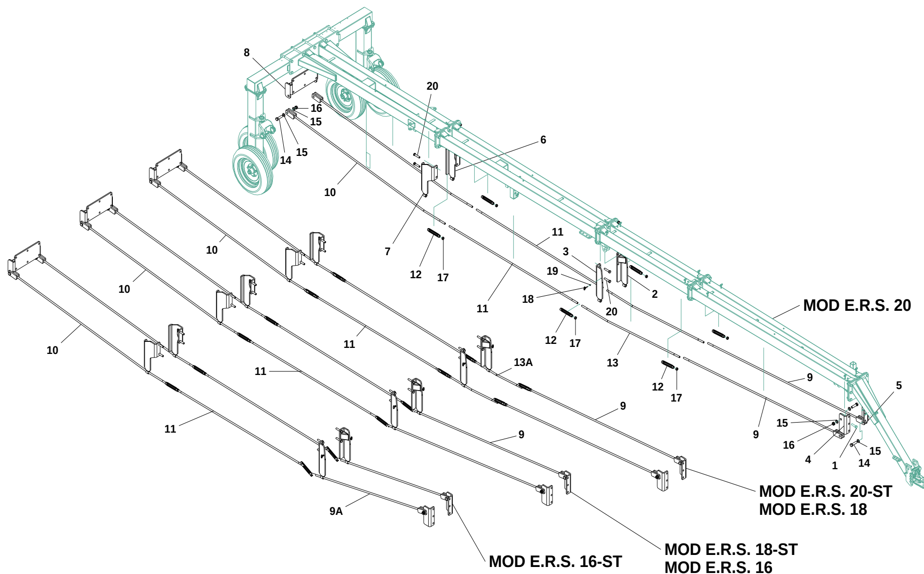
Tavola 20 - Table 20 - Planche 20 EASY RAKE SUPER STAR 16-18-20 / EASY RAKE SUPER STAR 16-18-20-22 AUTOSTERZ.-AUTOSTEER-AUTODIRECTEUR KIT TIRANTI – KIT TIE ROADS – KIT TIRANTS
