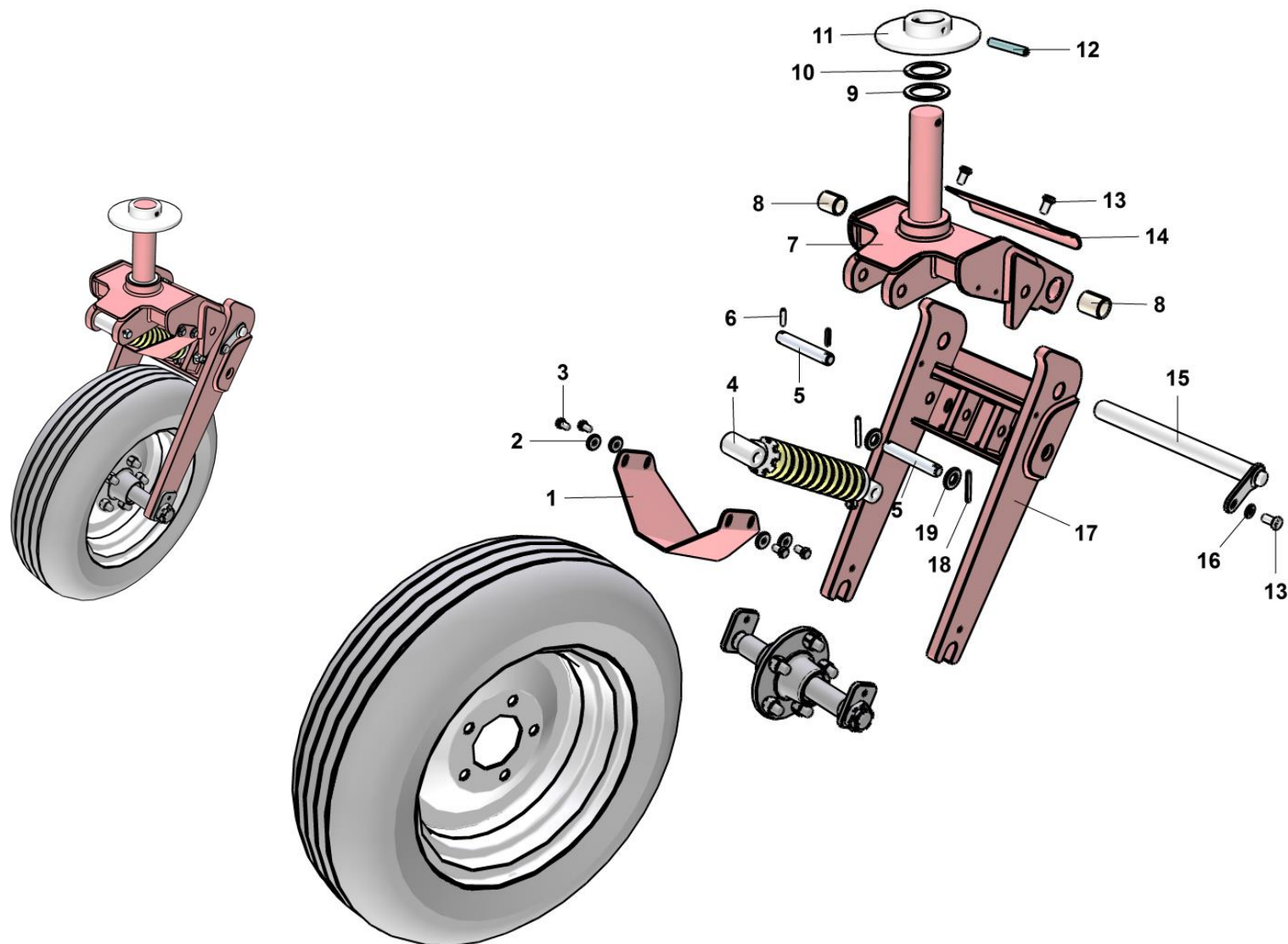
Tavola 22 - Table 22 - Planche 22 (OPTIONAL) EASY RAKE SUPER STAR 16-18-20 / EASY RAKE SUPER STAR 16-18-20-22 AUTOSTERZ.-AUTOSTEER-AUTODIRECTEUR
