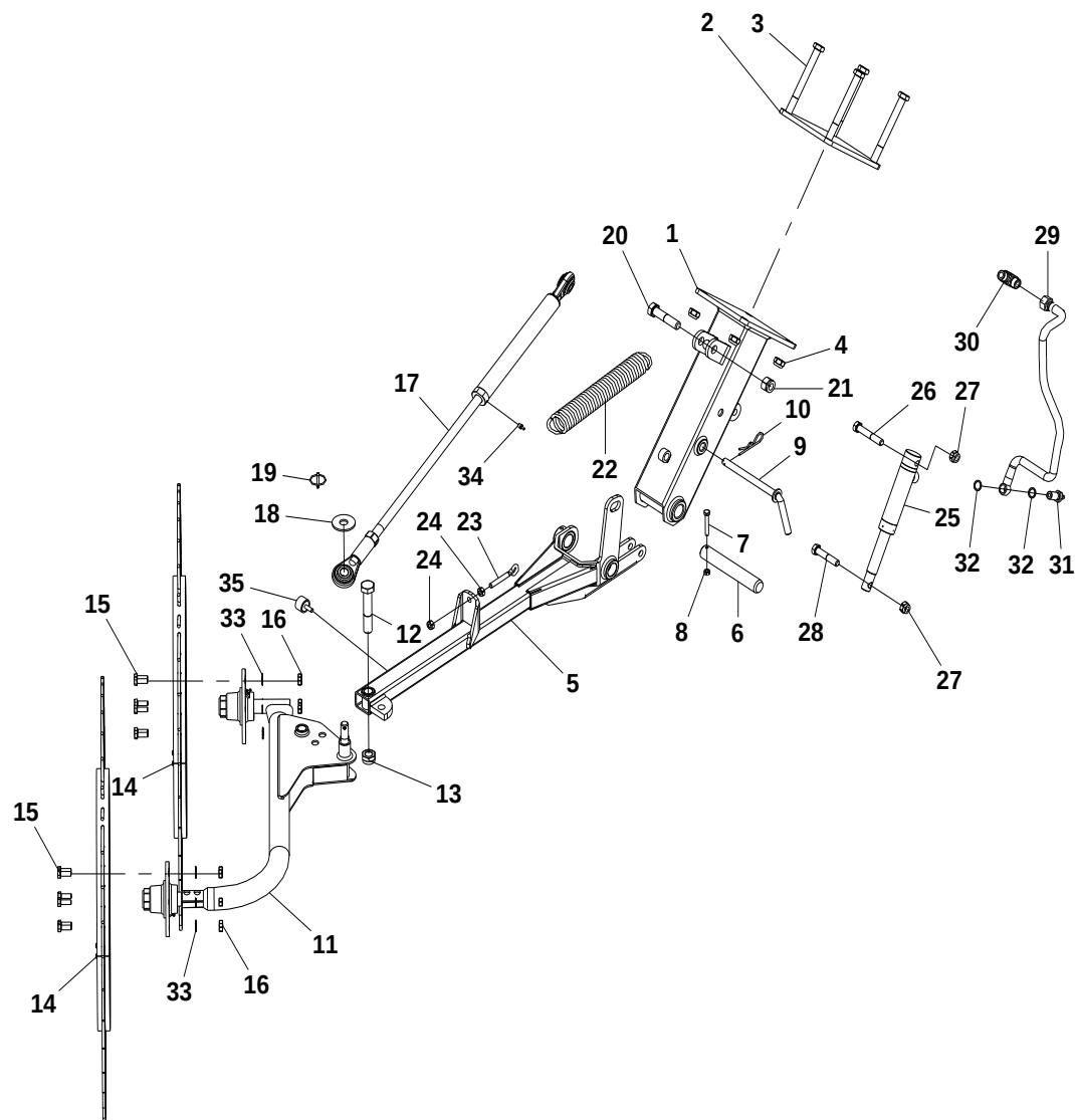
Tavola 16-Table 16-Planche 16- (OPTIONAL) - EASY RAKE SUPER STAR 16-18-20 / EASY RAKE SUPER STAR 16-18-20-22 AUTOSTERZ.-AUTOSTEER-AUTODIRECTEUR
